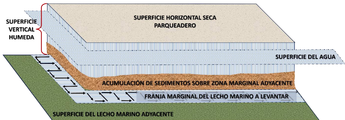
Imagen 3: Indicación de las superficies horizontal y verticales a inspeccionar. Cabe resaltar la franja del lecho marino, de 5 metros de ancho, a levantar batimétricamente
