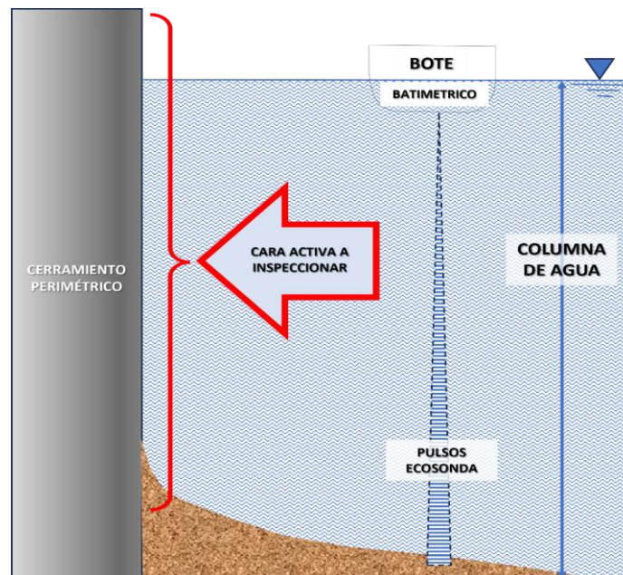
Ilustración 4: Esquema conceptual del levantamiento batimétrico de la franja de lecho marino
